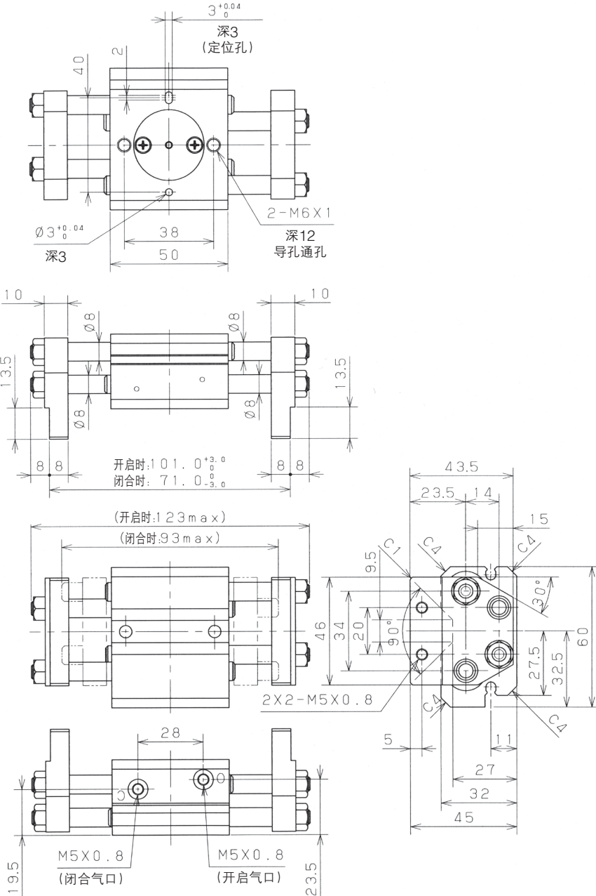
外形尺寸图 HP08-16
