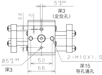
外形尺寸图 HP08-25
