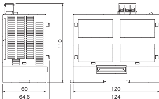
WJM 本体
