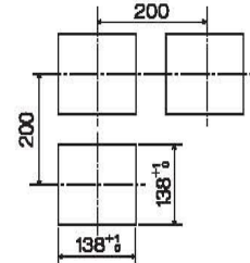
仪表屏开孔尺寸及最小间距
