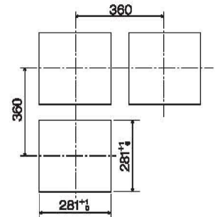
仪表屏开孔尺寸及最小间距
