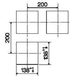
仪表屏开孔尺寸及最小间距
